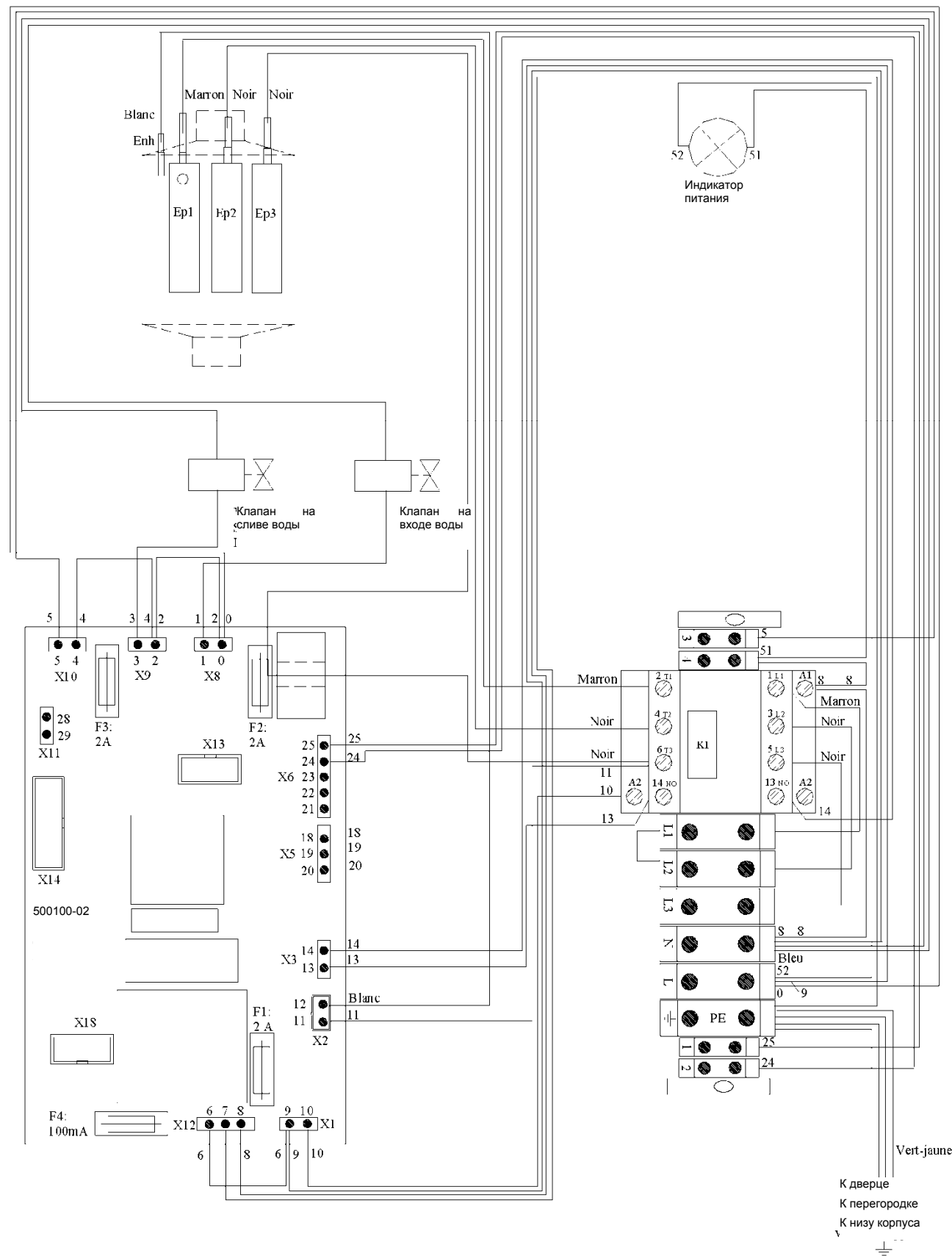
Схема электрических соединений SHE 5
