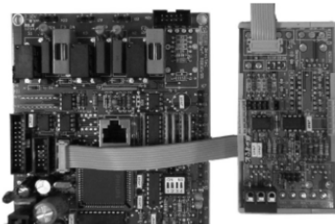
Плата 500800/01
