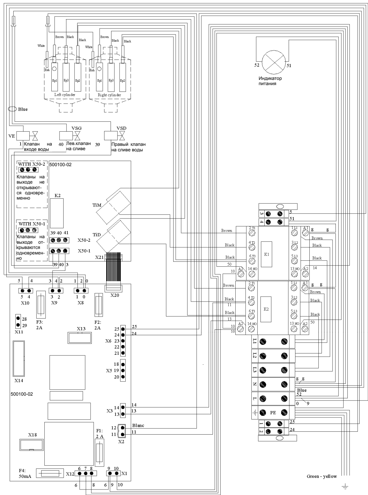
Схема электрических соединений SHE от 30 до 40 - 3×208–230 В, SHE от 40 до 60 - 3×380–690 В
