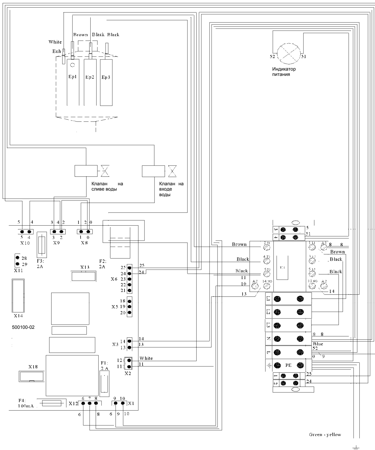
Схема электрических соединений SHE от 5 до 25 - 3×208–230 В, SHE от 5 до 30 - 3×380–690 В
