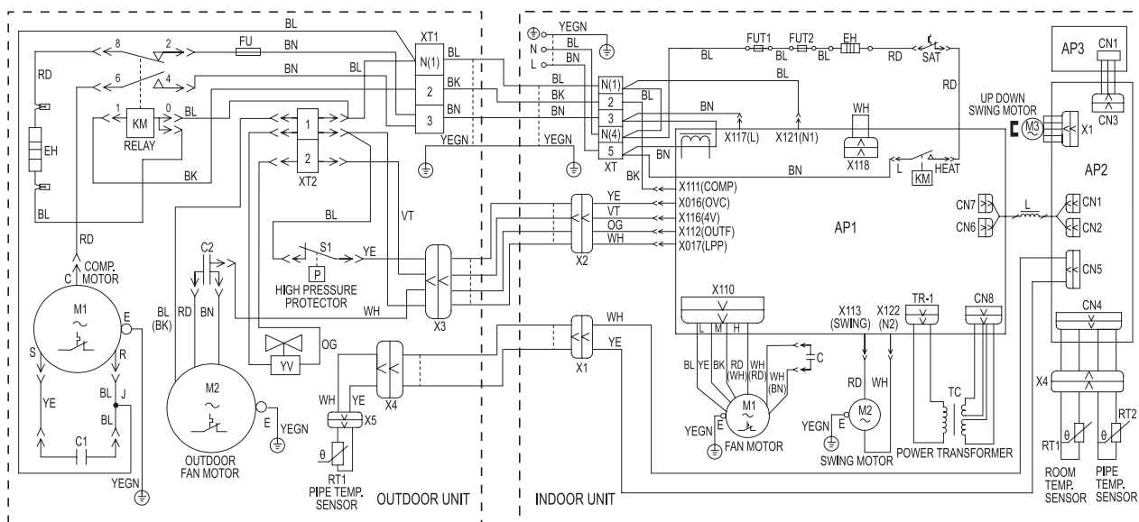
Схема электрическая модели GVHN24A1NK3AA
