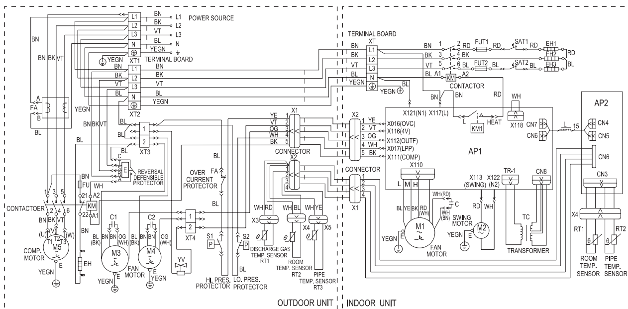
Схема электрическая модели GVHN42A2NM3AA
